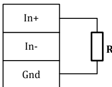
Измерение сопротивления 2-х проводная схема
